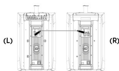
EVOX JMIX8 + EVOX J8 (stereo output)
